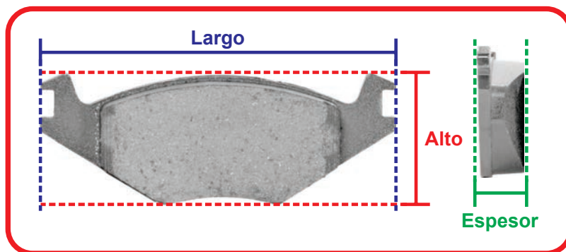
Manera de medir las Balatas de Disco
